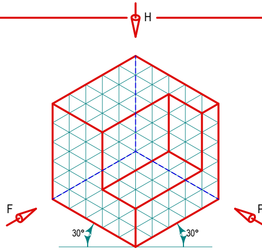
ISOMETRÍA
