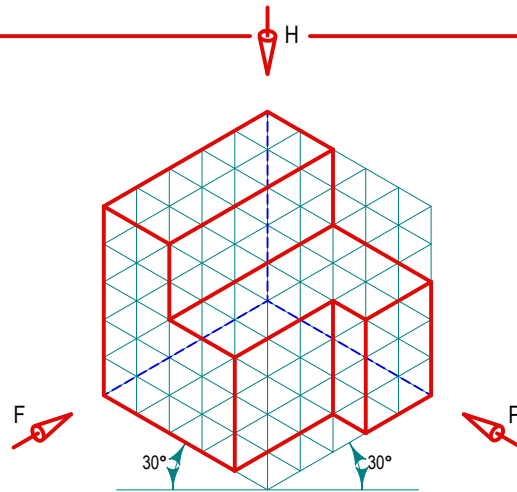
ISOMETRÍA
