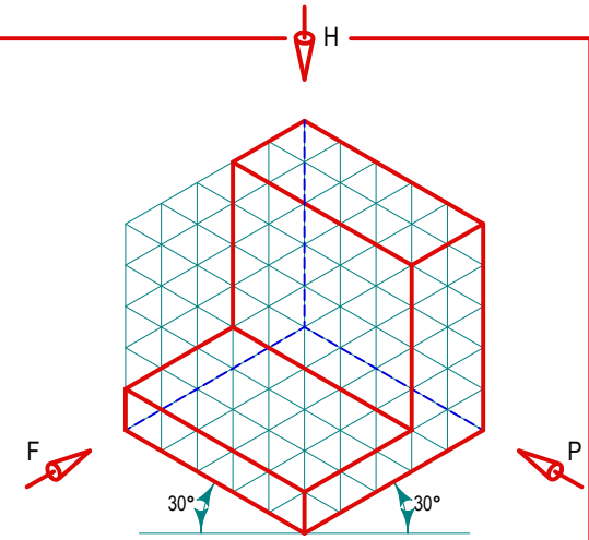
ISOMETRÍA
