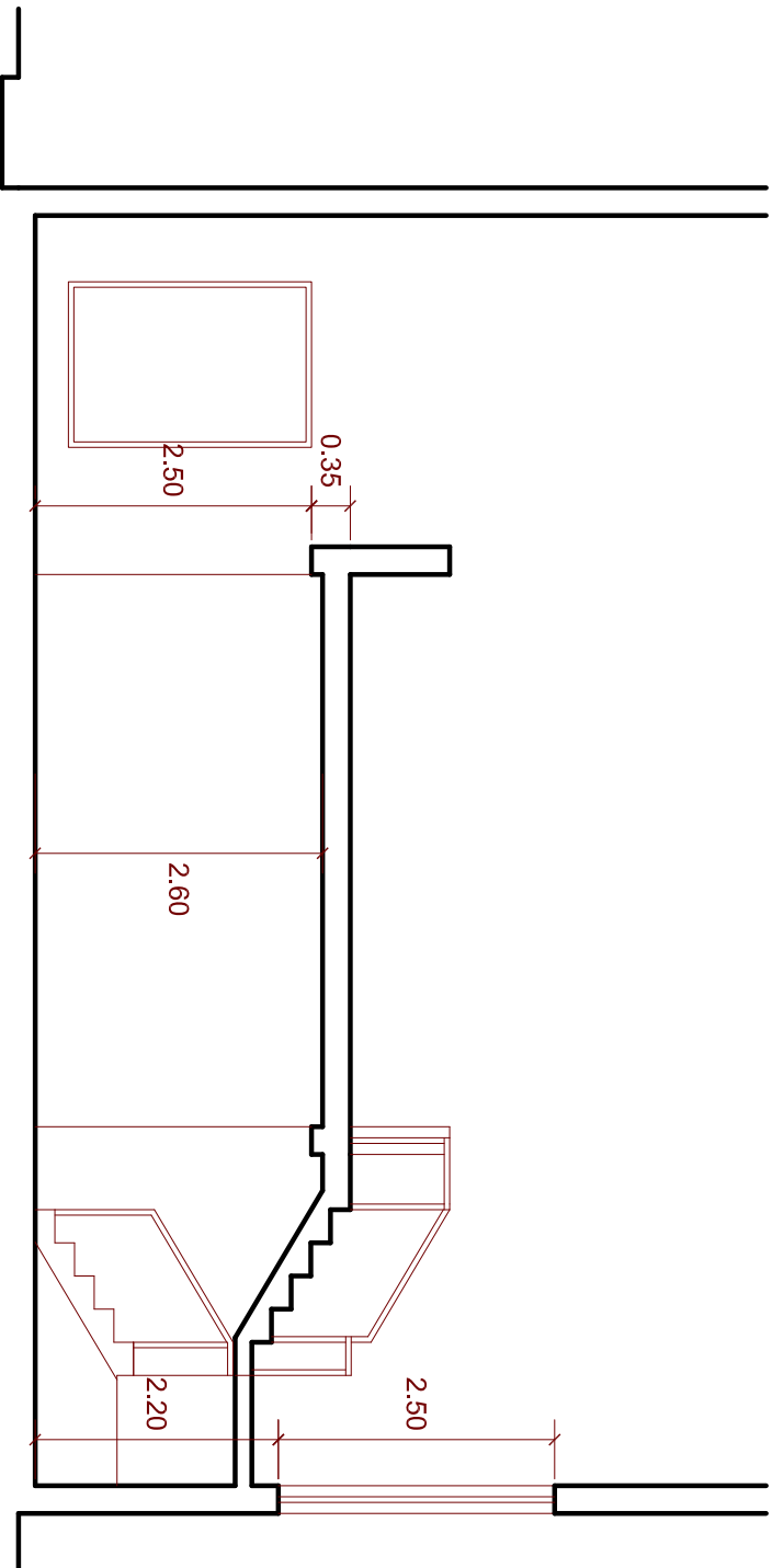
CORTE B-B' ESCALA: 1/75
